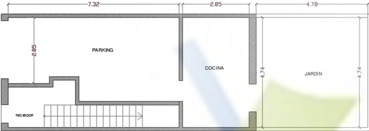
PLANTA BAJA
