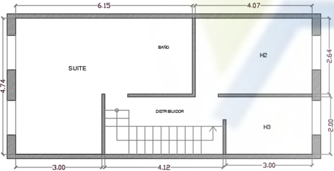
PLANTA SEGUNDA
